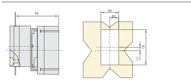
Разметка панели ( для выключателей стационарного и втычного исполнения )
