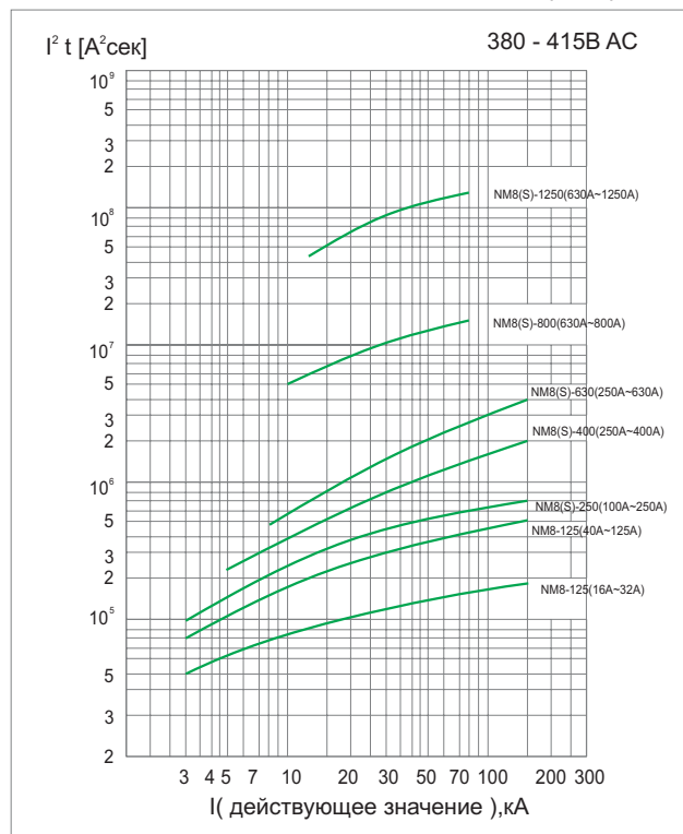
A^2сек характеристика
